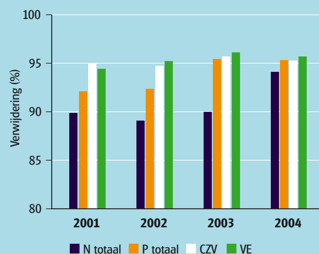
Figuur 2: Verwijderingsrendementen AWZI Schiphol
